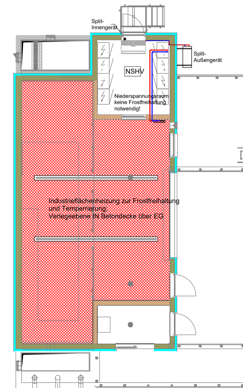
Grundriss EG Ind.FBH
