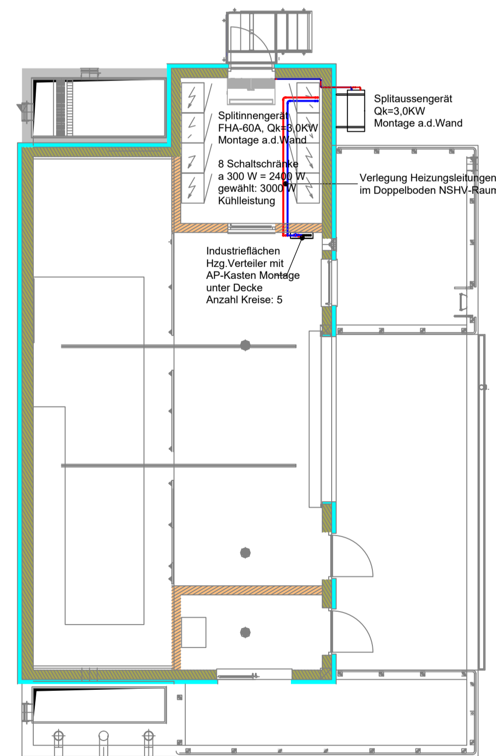
Grundriss EG
